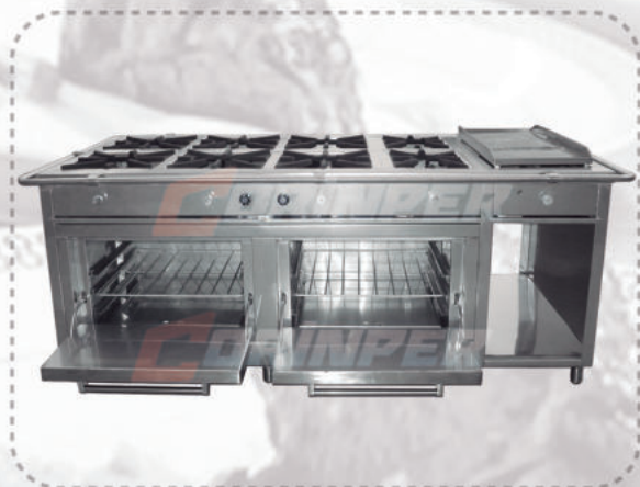
006 COCINA INDUSTRIAL CENTRAL ( 8 Hornillas , Plancha Freidora y 2 Hornos )
